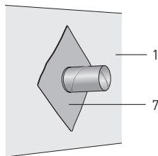
Genomföring tätas med Halotex Rörmanschett eller Halotex Byggtätningstejp.
