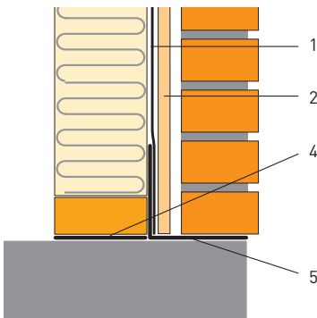
Anslutning mot tegelfasad.
