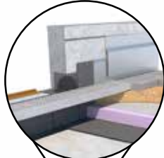
Anslutning till vertikal yta vid tröskel
