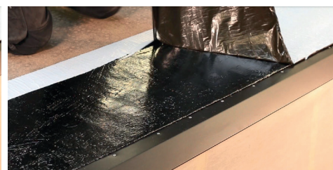
6. Dra bort releasefilmen på den del som hamnar på takytan, lämna tills vidare kvar releasefilmen på den del som hamnar över fotplåten. På så vis undviker man att tätskiktet klistrar fast på fotplåten innan man riktat in remsan.
