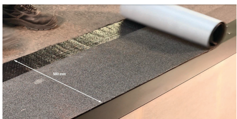
4. Anslutning mot fotplåten görs med max 500 mm bred remsa av E-Lit LA. Alternativt dras våderna ända ner mot fotplåten.
